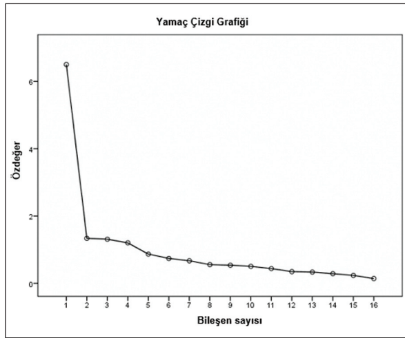
ŞEKİL 1: Klostrofobi Ölçeği yamaç çizgi grafiği
