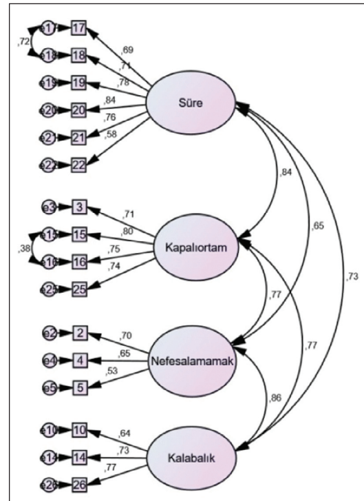
ŞEKİL 2: Klostrofobi Ölçeği doğrulayıcı faktör analizi modeli (n=127)
