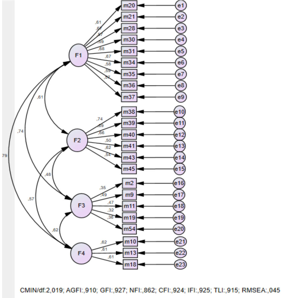
Görsel 1 DFA yol diyagramı
