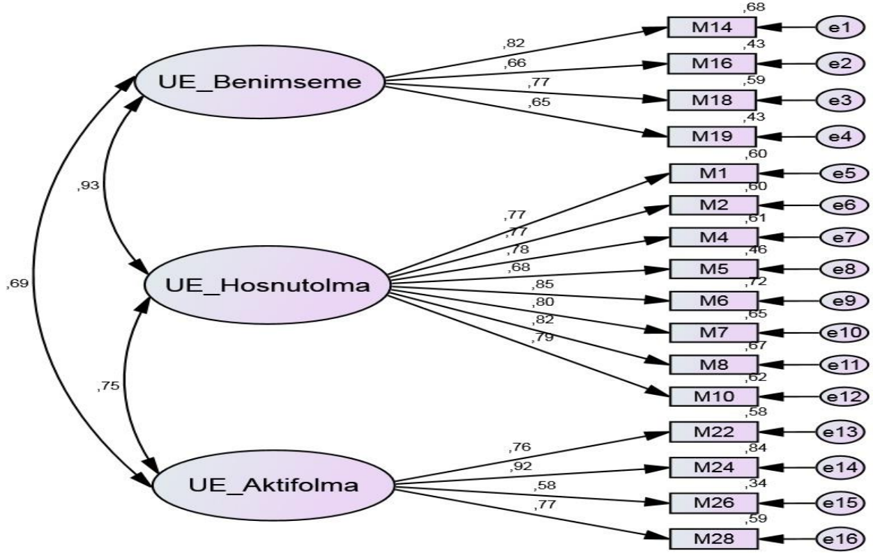
Şekil 1. Doğrulayıcı faktör analizi ölçek yapısı
