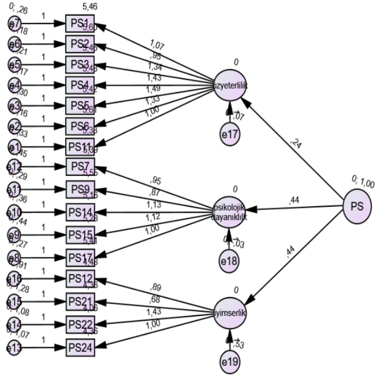
Şekil 1. Psikolojik Sermaye DFA Diyagramı
