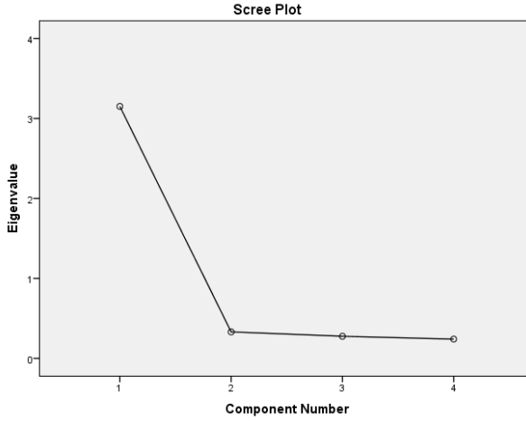
Şekil 1. Modele İlişkin Yamaç Çizgi Grafiği
