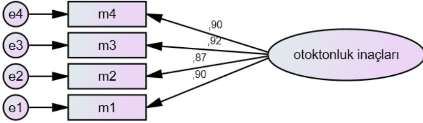
Şekil 2: OİÖ Doğrulayıcı Faktör Analizi Path Diyagramı
