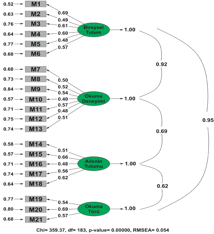
Şekil 2. Yol analizi
