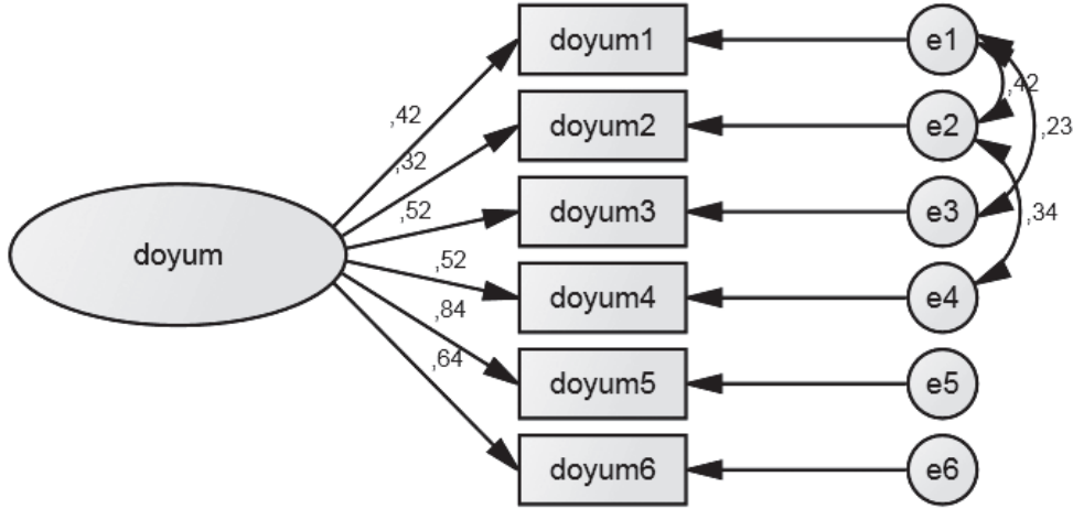
Şekil 2. Fedakarlık Doyum Ölçeği için Modifiye Edilmiş Tek Faktörlü Model
