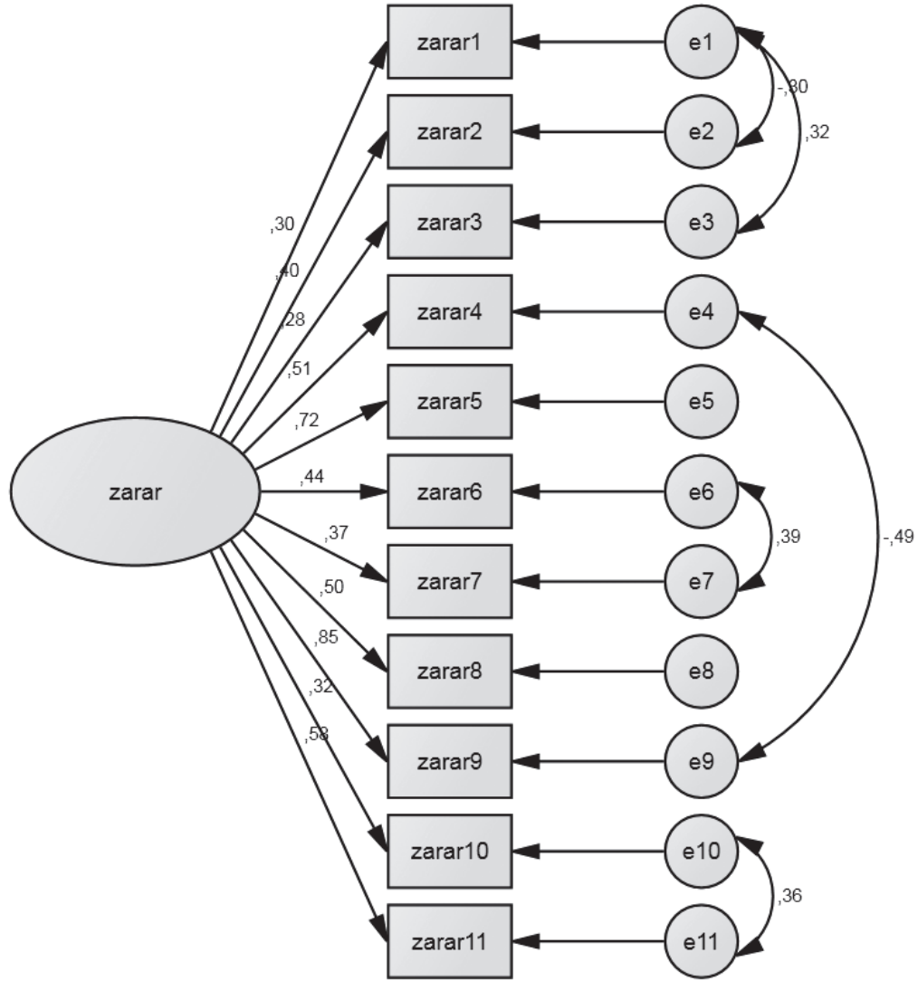
Şekil 1. Fedakarlıkta Algılanan Zarar Ölçeği için Modifiye Edilmiş Tek Faktörlü Model
