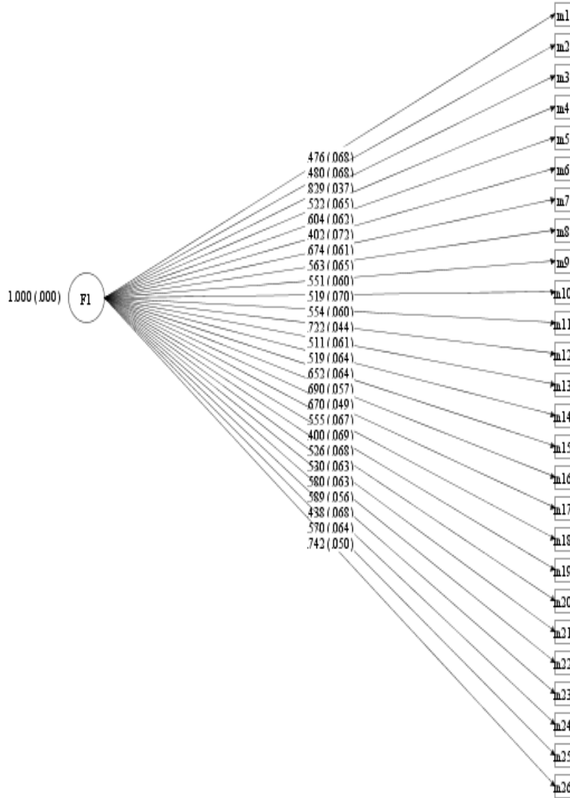
Şekil 1. Evlilik Değerleri Ölçeğinin Doğrulayıcı Faktör Analizi Modeli
