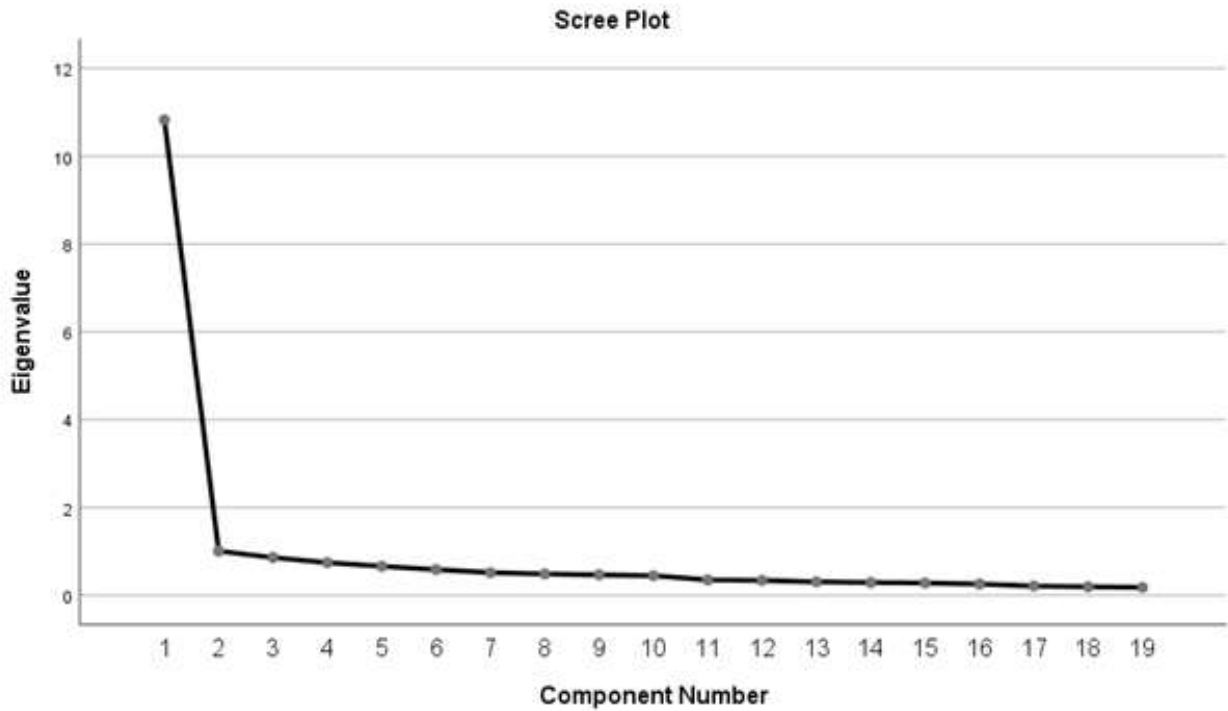
Şekil 2. Scree Plot Grafiği
