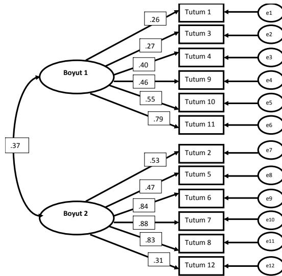
Şekil 2. Aldatmaya Yönelik Tutum Ölçeği için İki Boyutlu DFA Modeli
