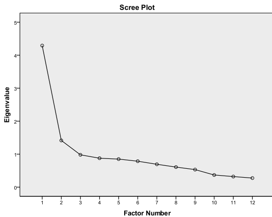
Şekil 1. Çizgi (Scree Plot) Grafiği
